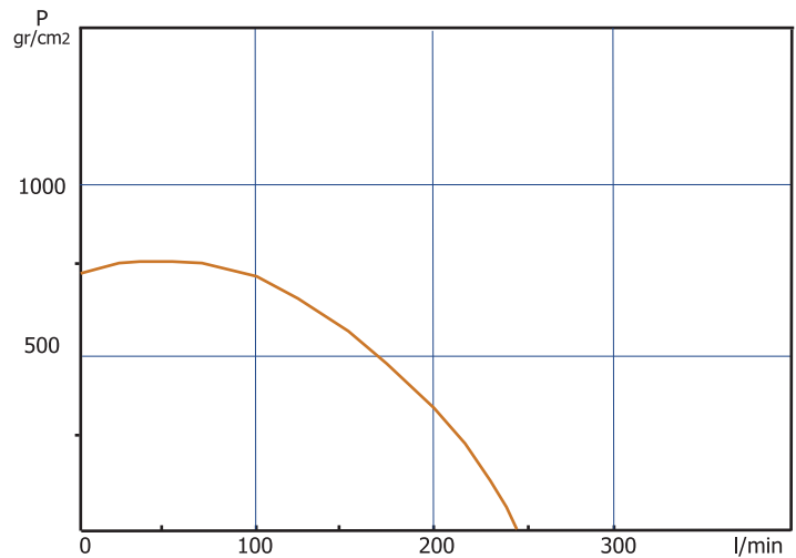
CURVA HIDRAULICA
